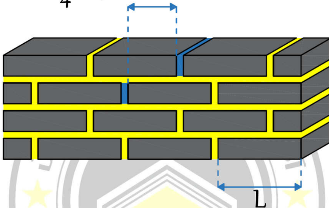
شکل ۱-۱۲ پیوند ممتد
