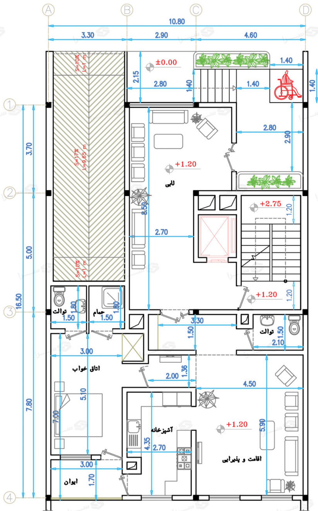
پلان طبقه همکف / طراحی: دکتر اکرم خدای مدرس دوره های طراحی نظام مهندسی ساختمان
