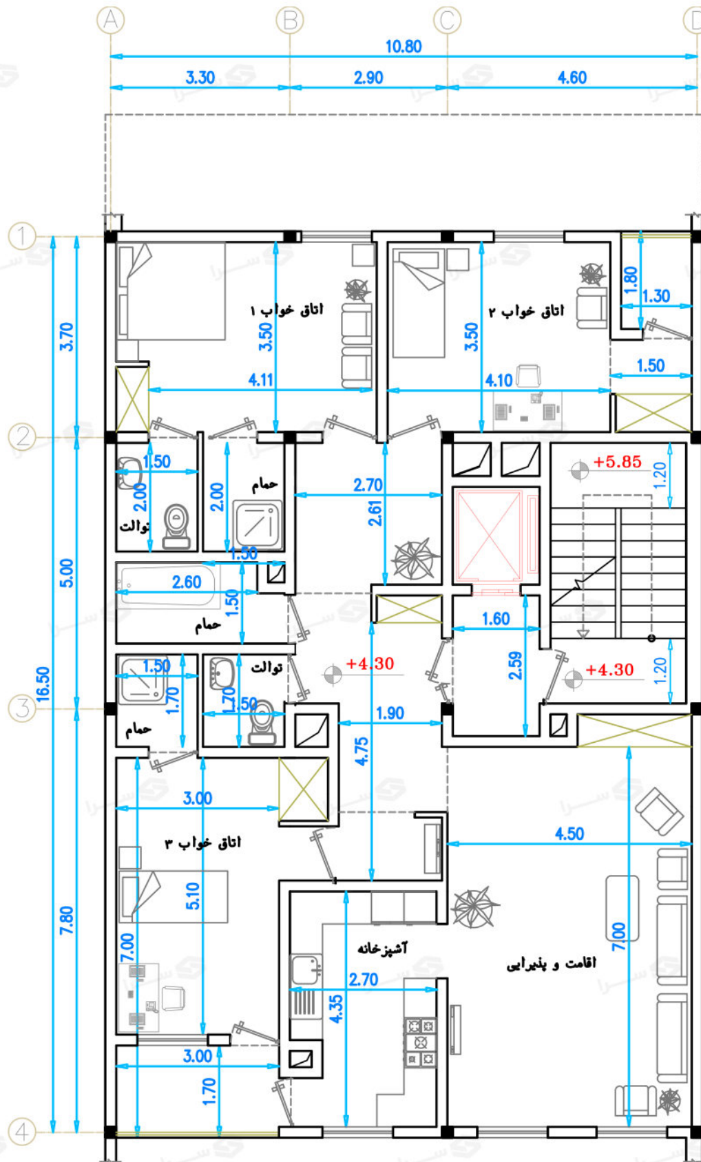
پلان طبقه اول / طراحی: دکتر اکرم خدای مدرس دوره های طراحی نظام مهندسی ساختمان
